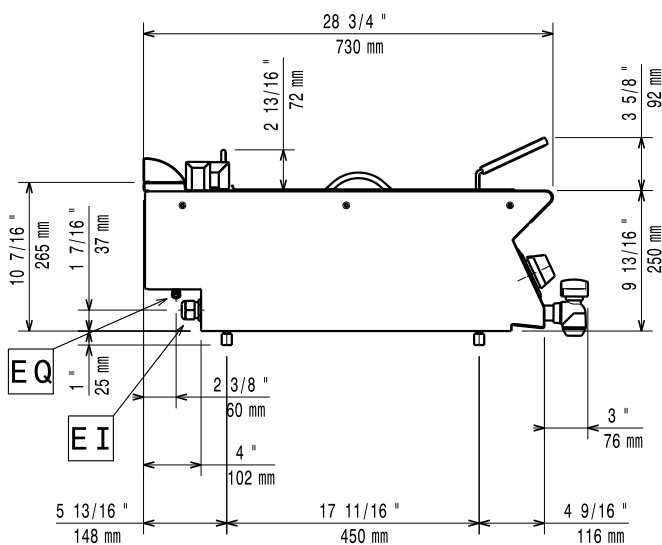
Sivulta
